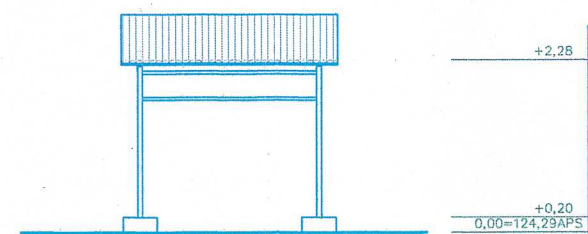
istočno pročelje
